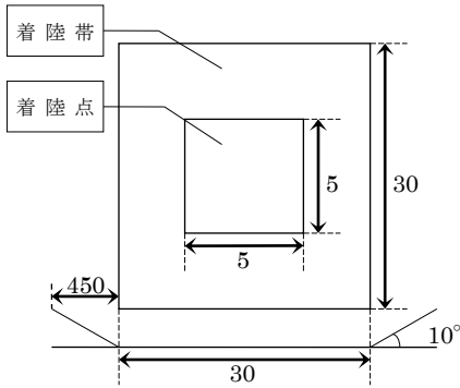
(a-1) 小型機(OH-6)の場合《標準》 単位：m
