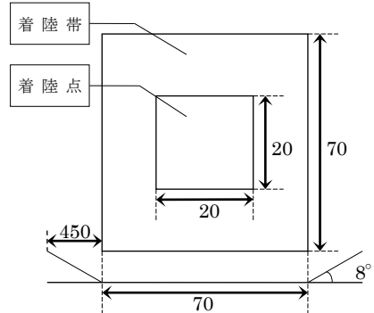
(d-2) 大型機(CH-47)の場合《応急》 単位：m
