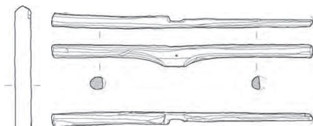
▲出土した杵の腕木実測図
