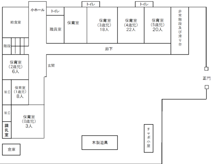
1階平面図
