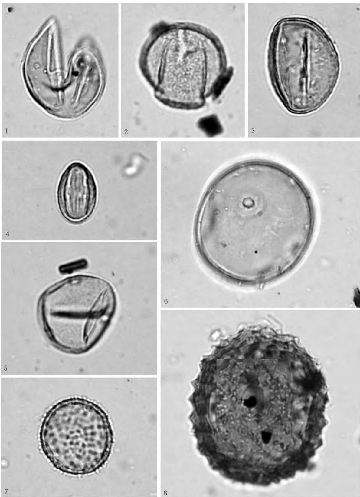
4—図版2 1d区の西側トレンチの2459から産出した花粉化石
