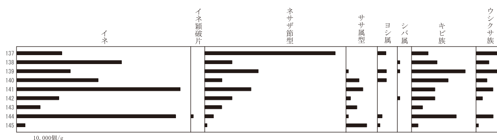
4-図4 下田南遺跡における植物珪酸体分布図
