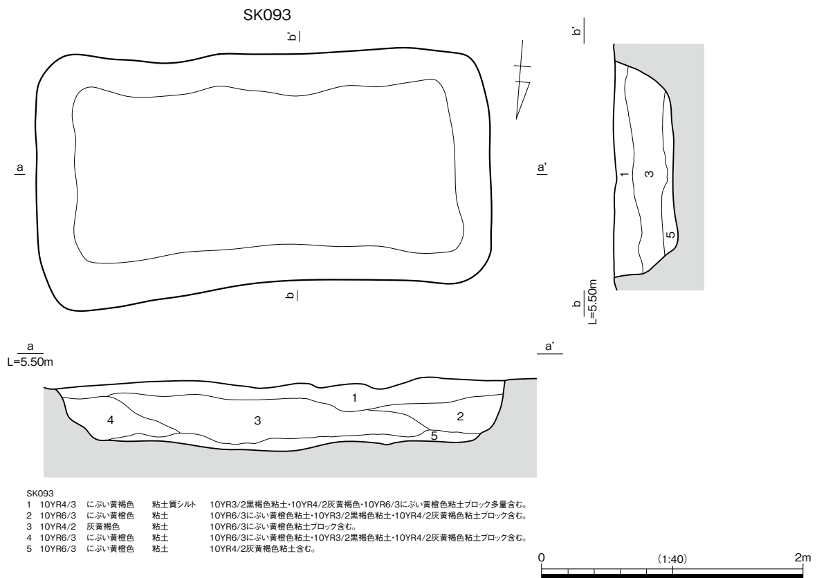
2d区 SK092・SK093 遺構図
