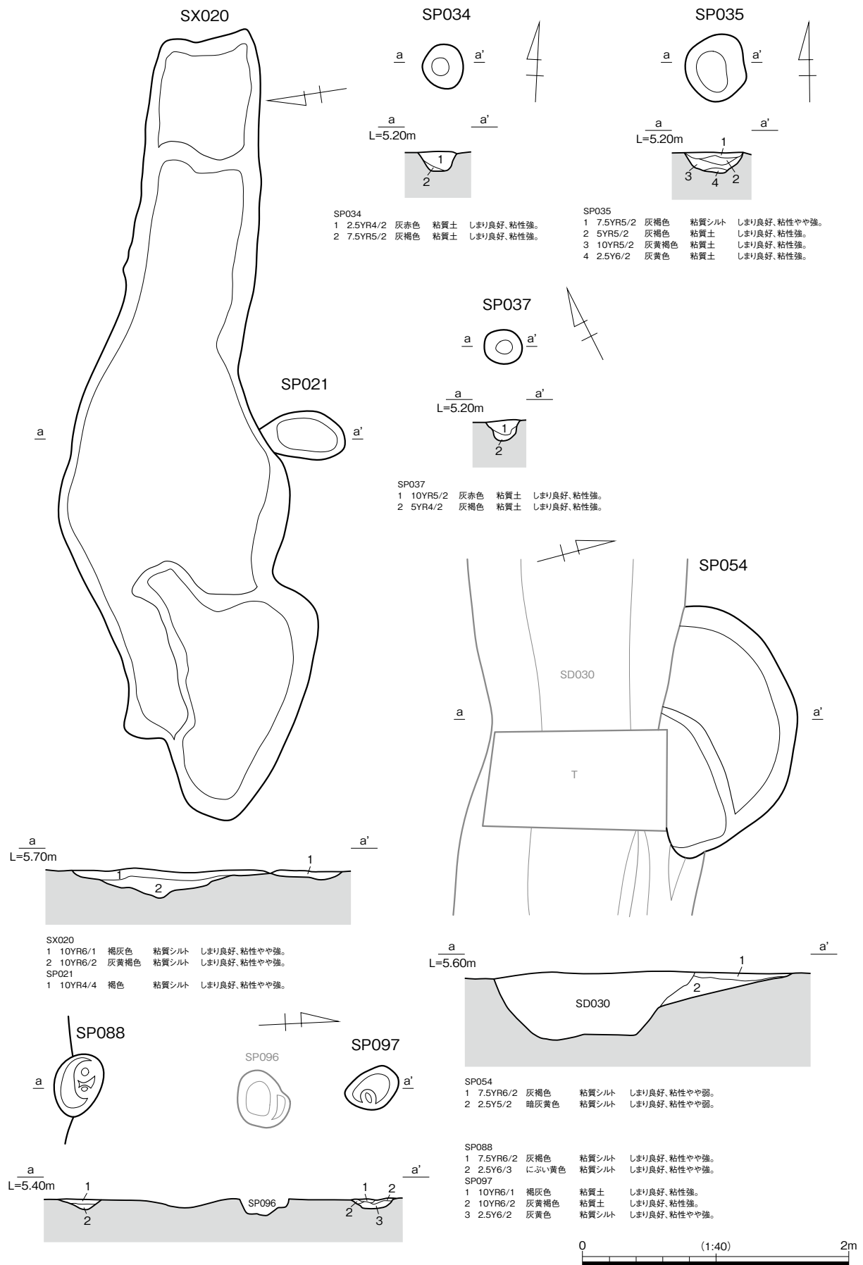
2e区1面 SP021・SP034・SP035・SP037・SP054・SP088・SP097・SX020 遺構図
