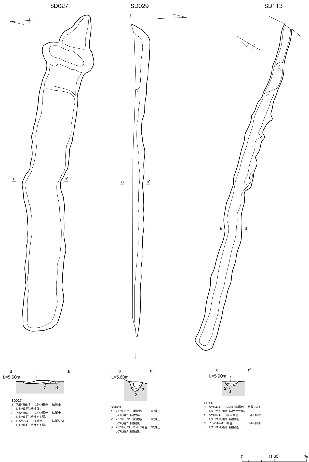
2e区1面 SD027・SD029・SD113 遺構図
