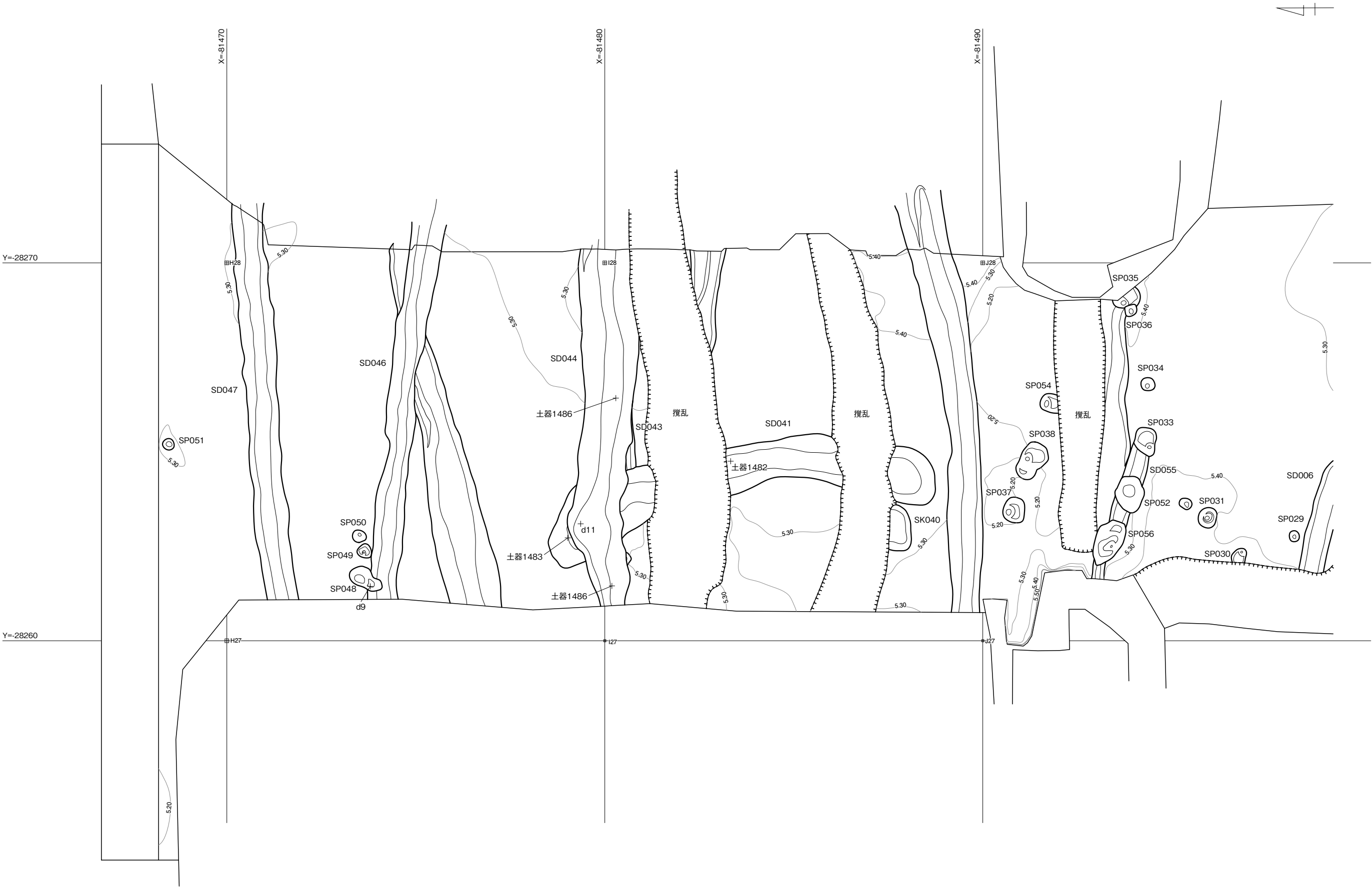
Rf区2面 遺構位置図(1)
