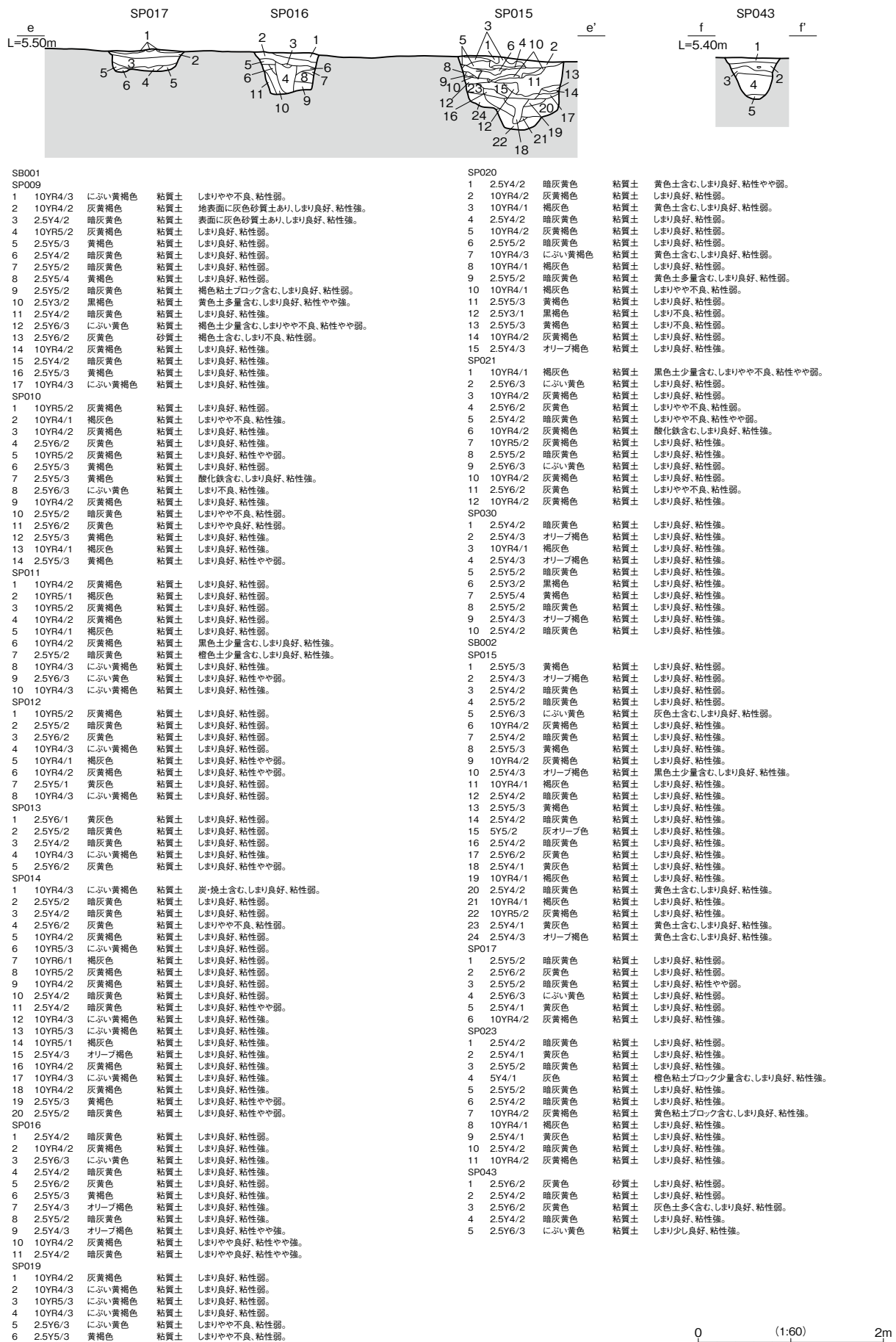
Rc区 SB001・SB002② 遺構図
