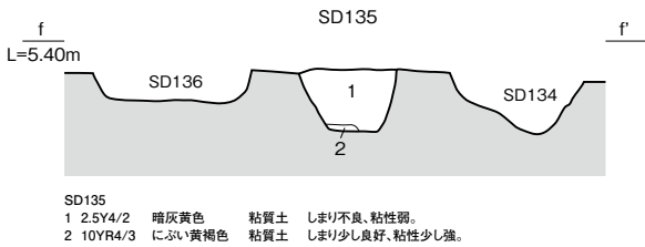
Ra区 SD001・SD097・SD135 遺構図
