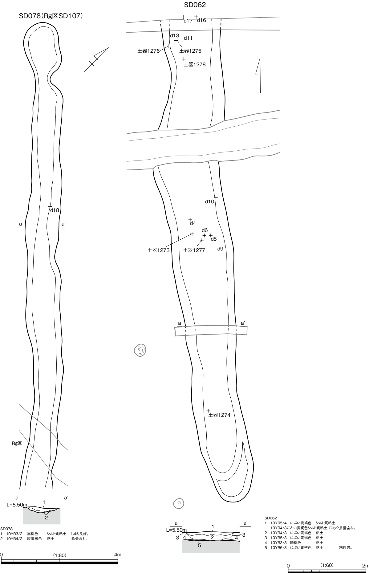
2d区 SD062・SD078 遺構図
