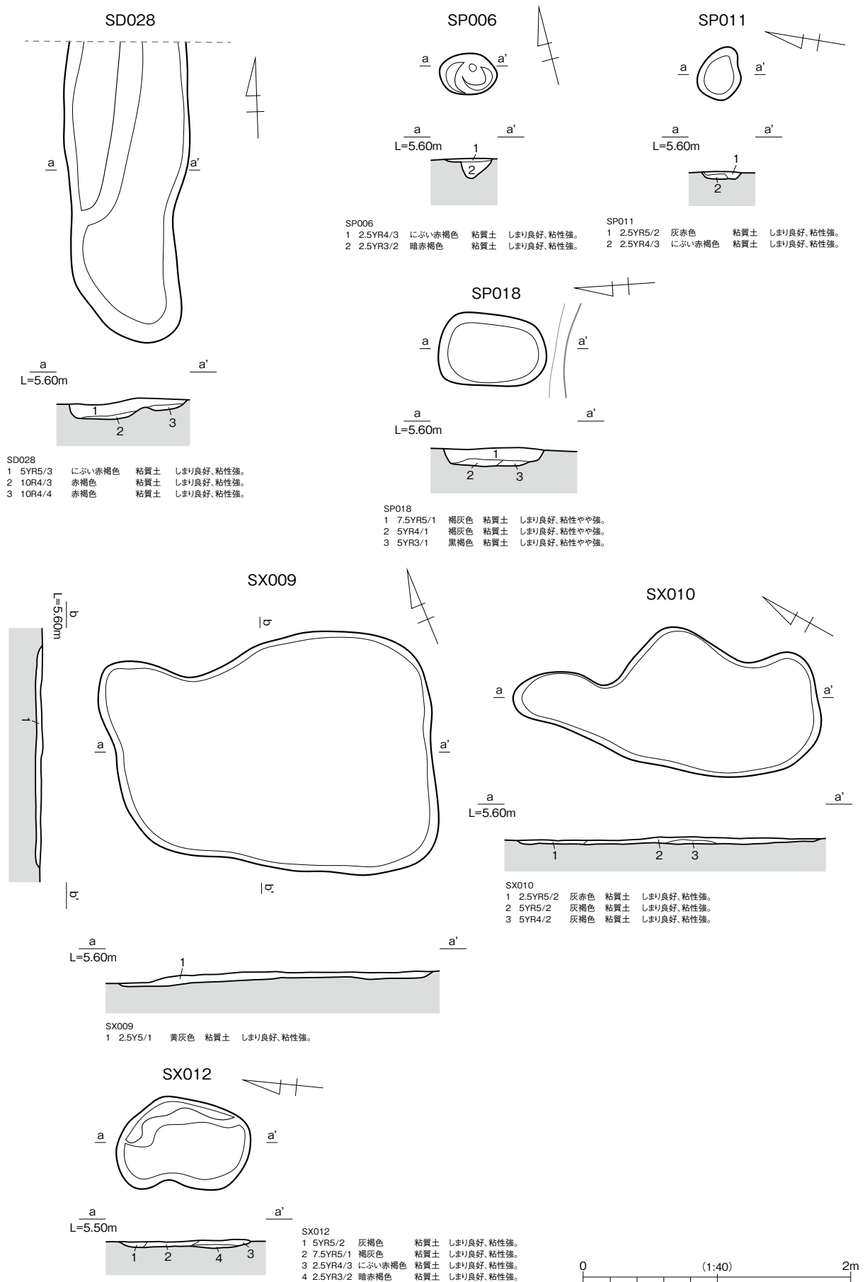
Rg区1面 SD028・SP006・SP011・SP018・SX009・SX010・SX012 遺構図
