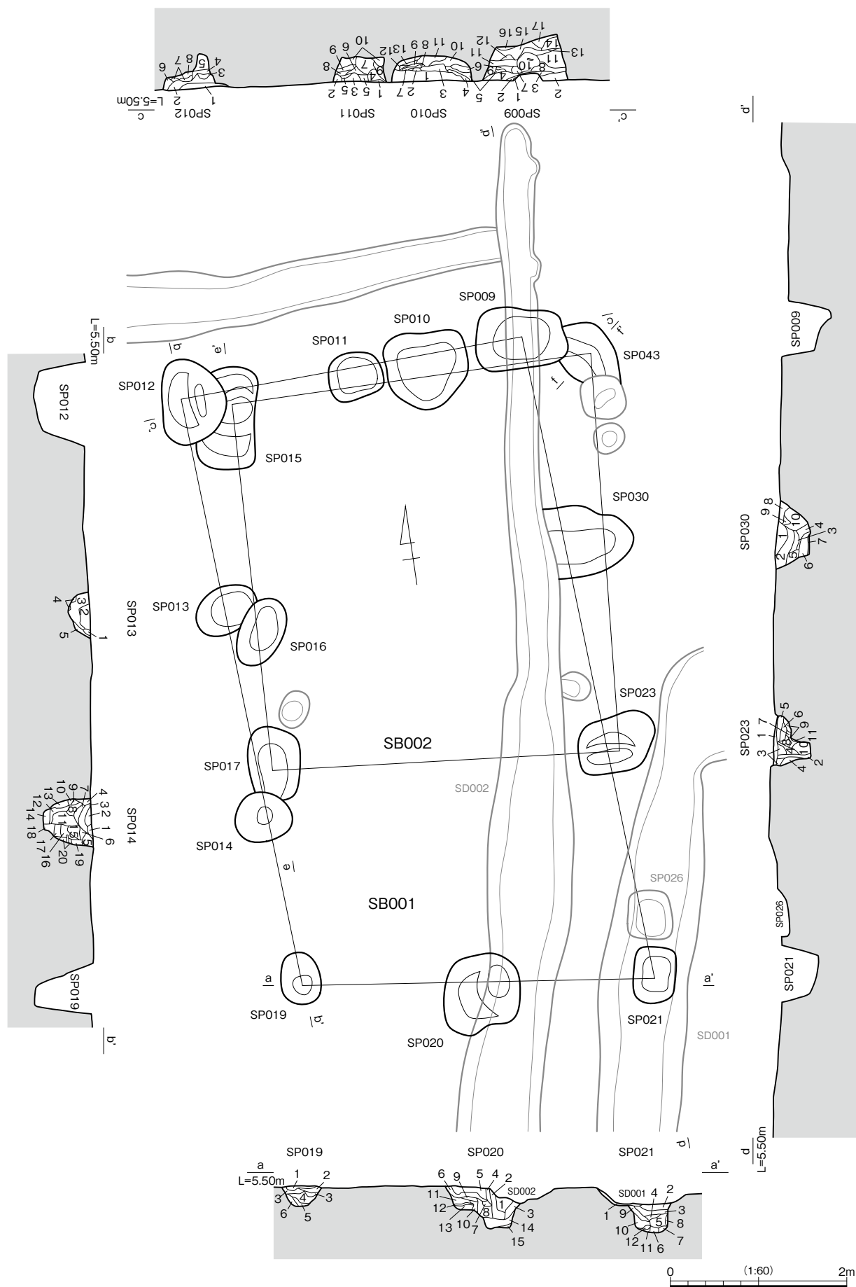
Rc区 SB001・SB002① 遺構図
