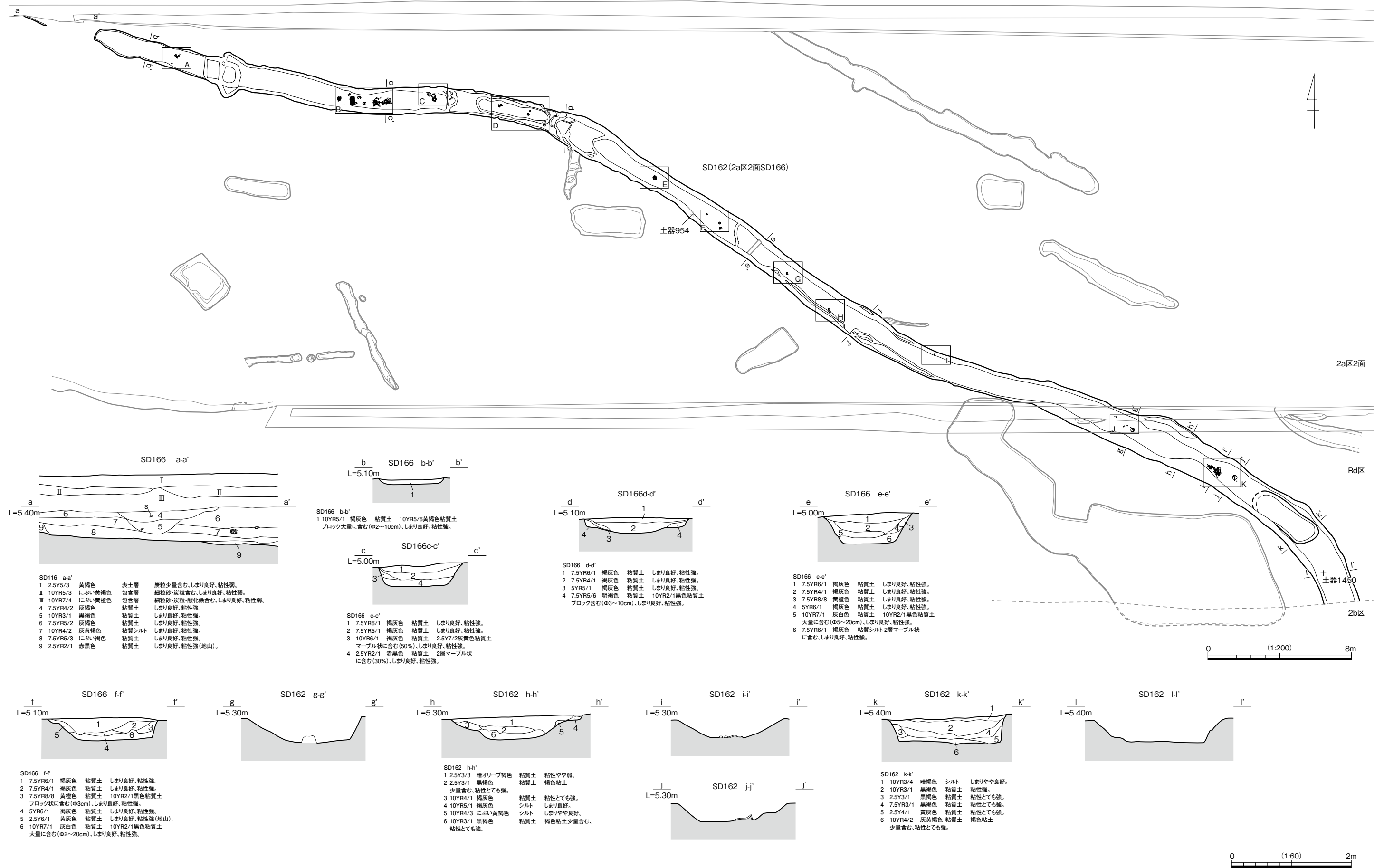
Rd区 SD162(2a区2面SD166) 遺構図
