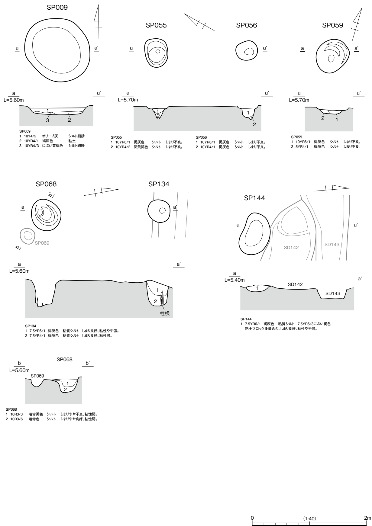
2a区1面 SP009・SP055・SP056・SP059・SP068・SP134・SP144 遺構図
