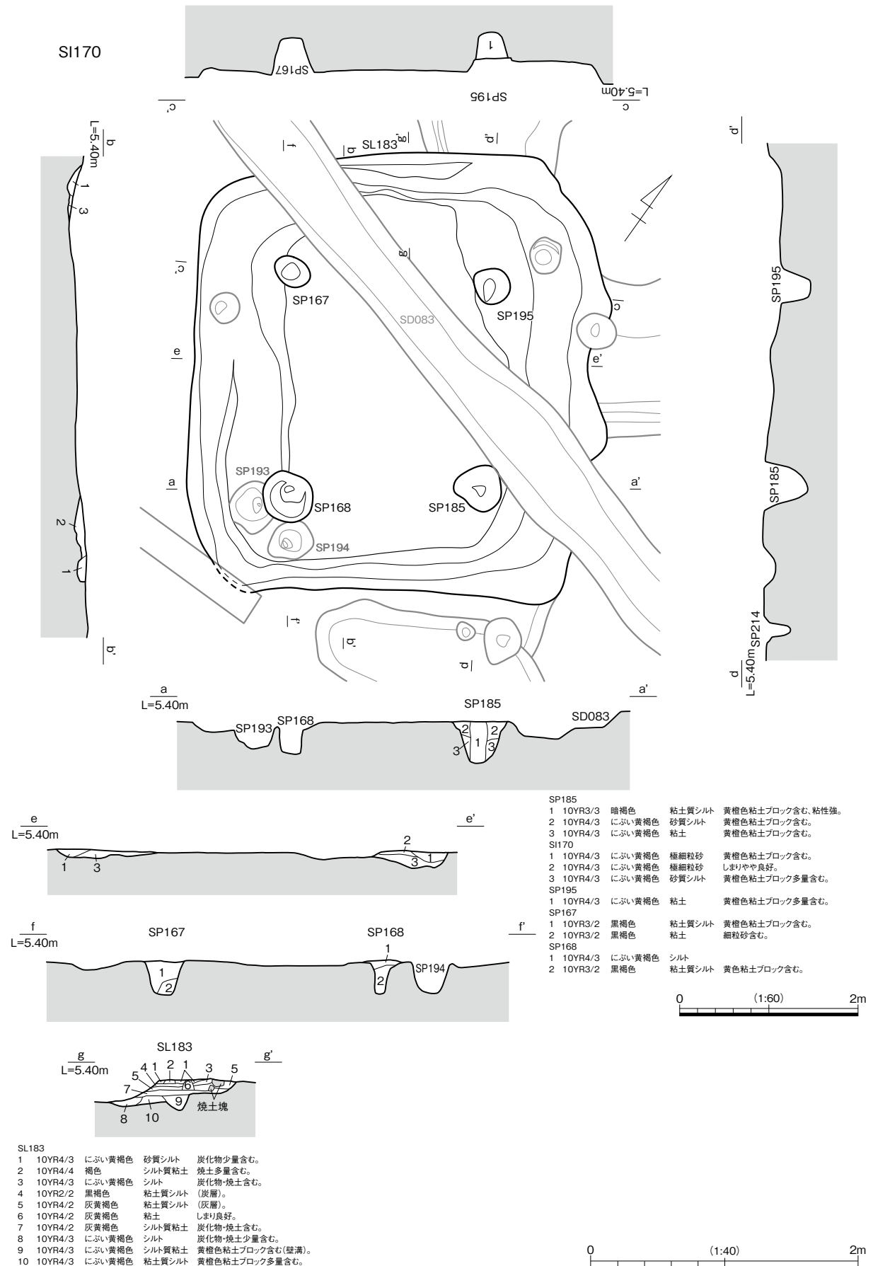
2b区 SI170 遺構図
