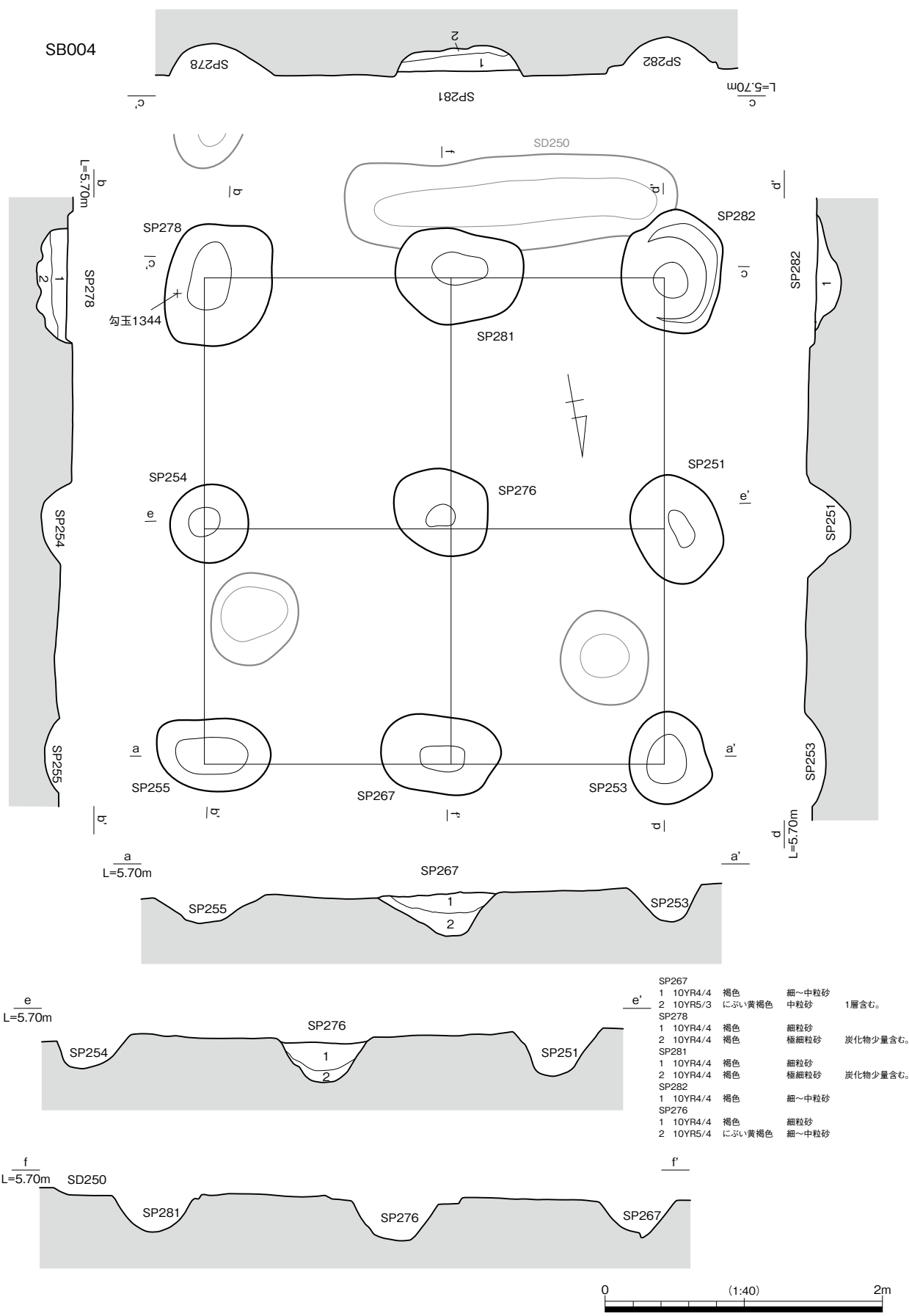
2b区 SB004 遺構図
