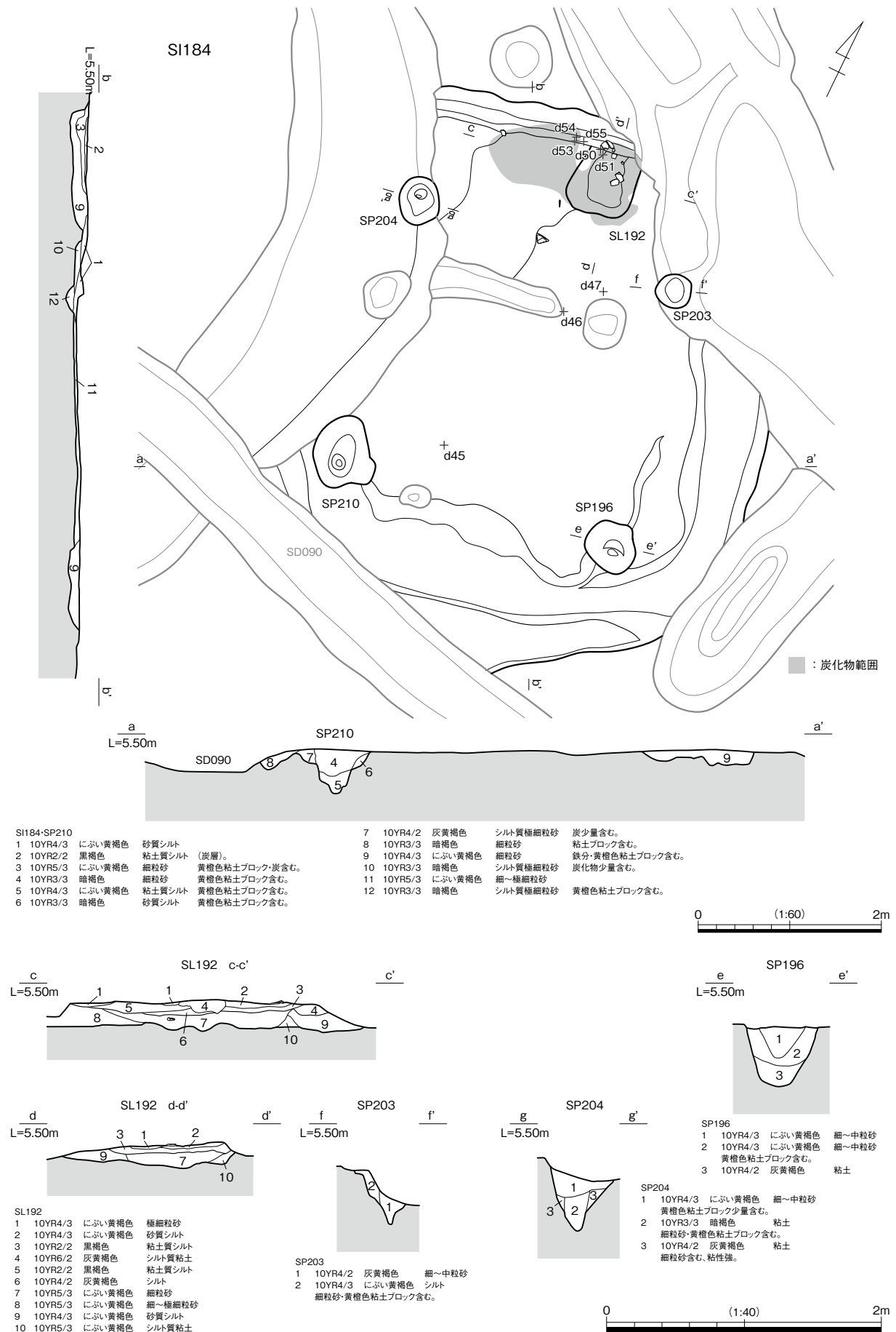
2b区 SI184 遺構図
