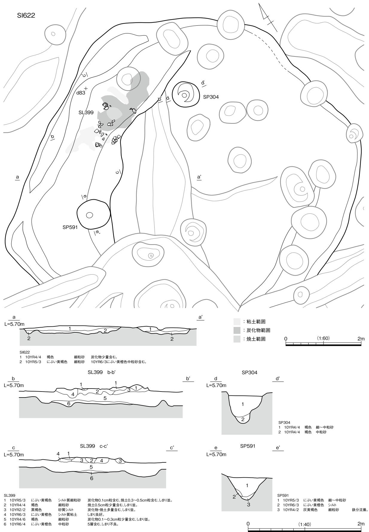
2b区 SI622 遺構図
