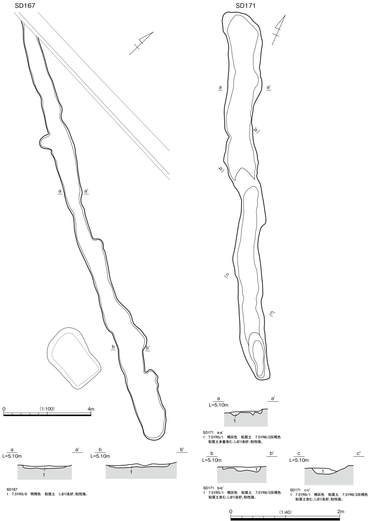
2a区2面 SD167・SD171 遺構図
