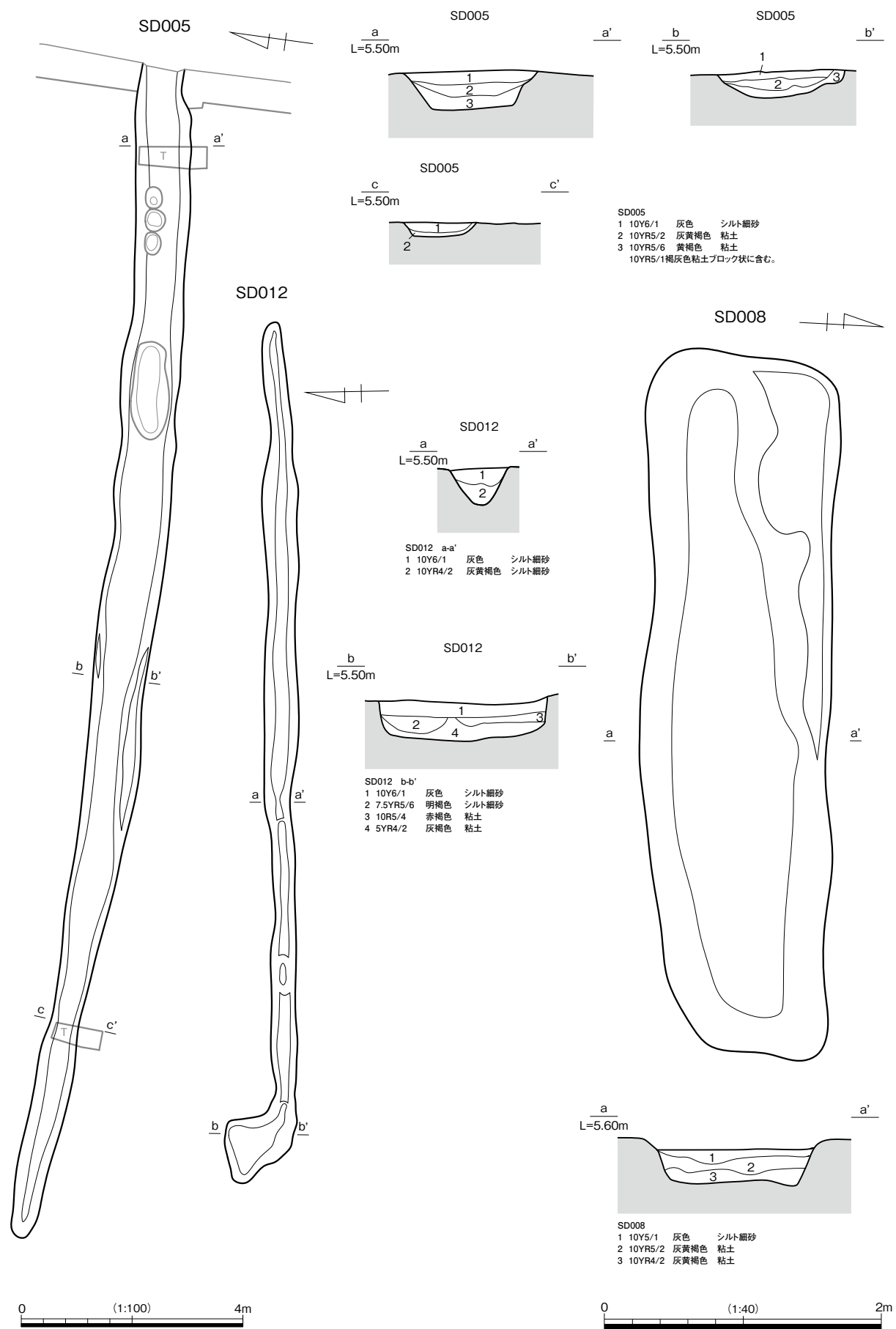
2a区1面 SD005・SD008・SD012 遺構図
