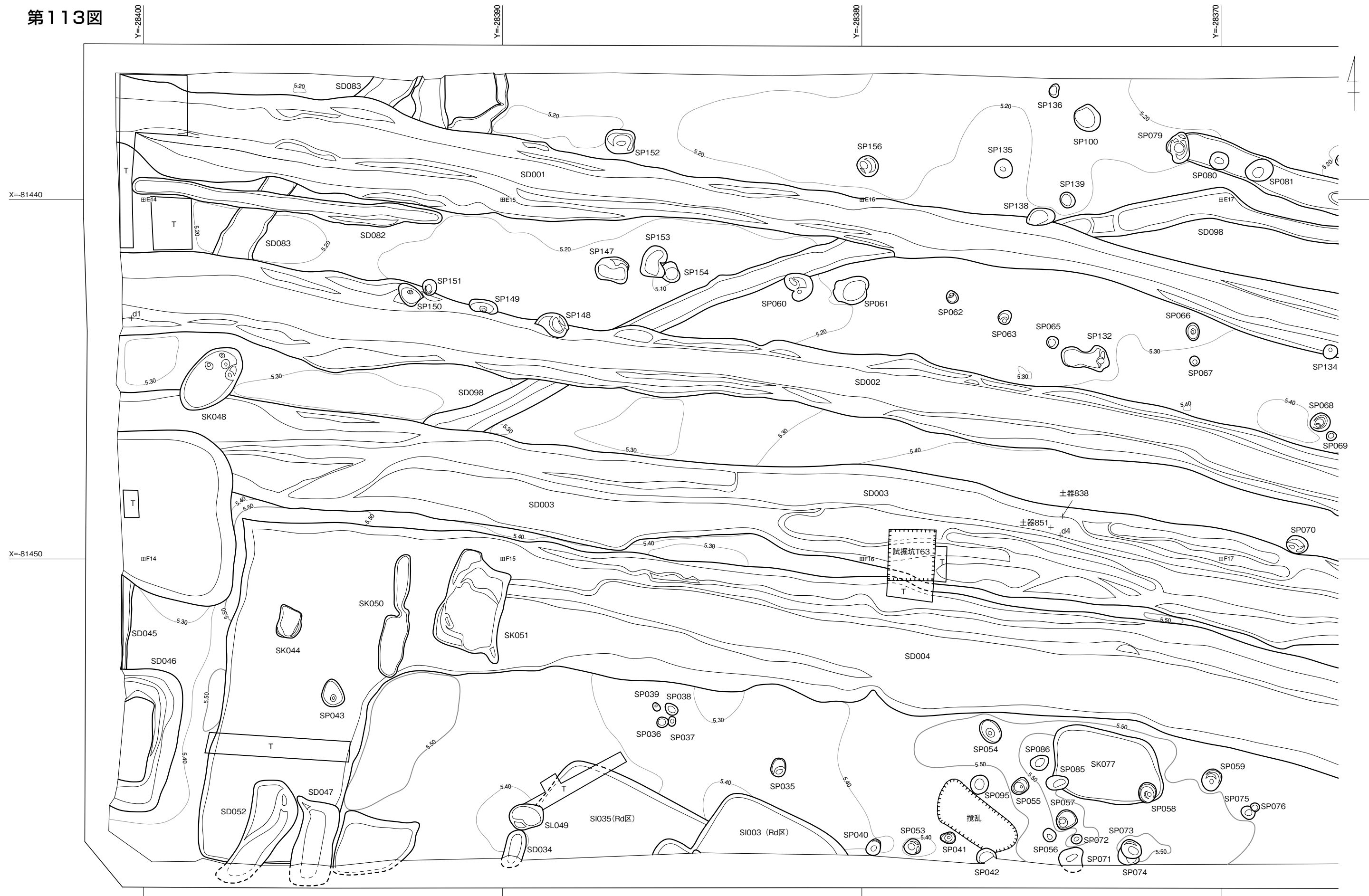
2a区1面 遺構位置図(1)
