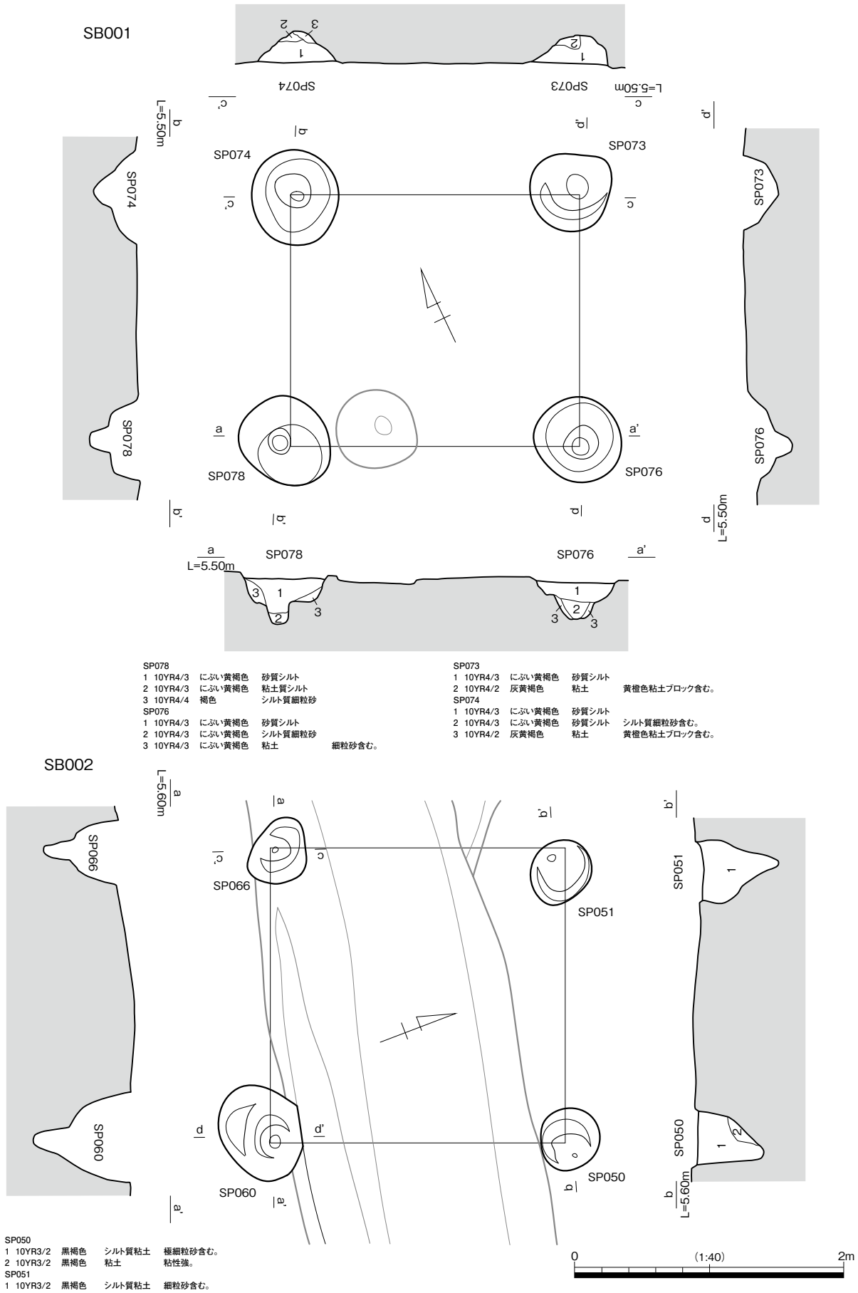
2b区 SB001・SB002① 遺構図
