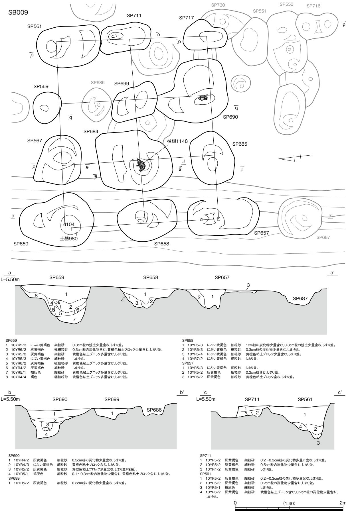
2b区 SB009① 遺構図
