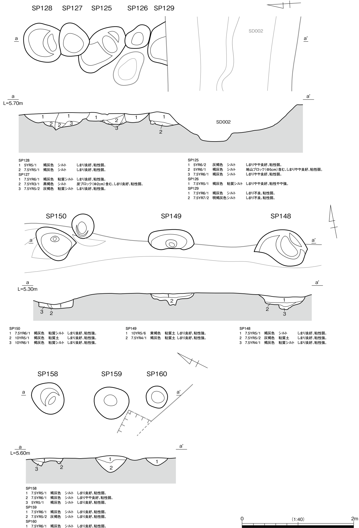
2a区1面 SP125～SP129・SP148～SP150・SP158～SP160 遺構図
