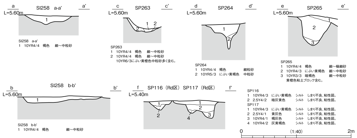
2b区 SI257②・SI258 遺構図
