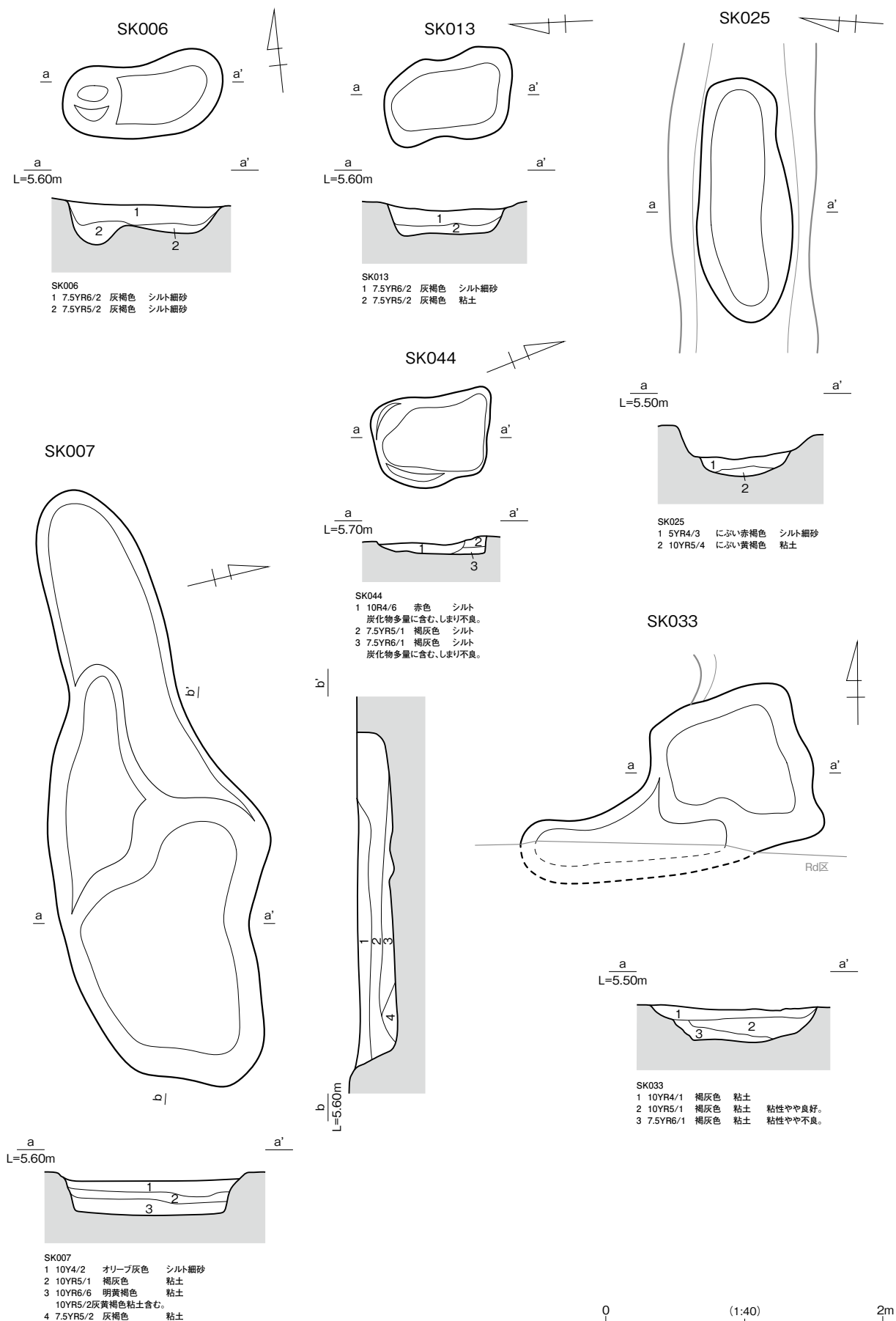
2a区1面 SK006・SK007・SK013・SK025・SK033・SK044 遺構図
