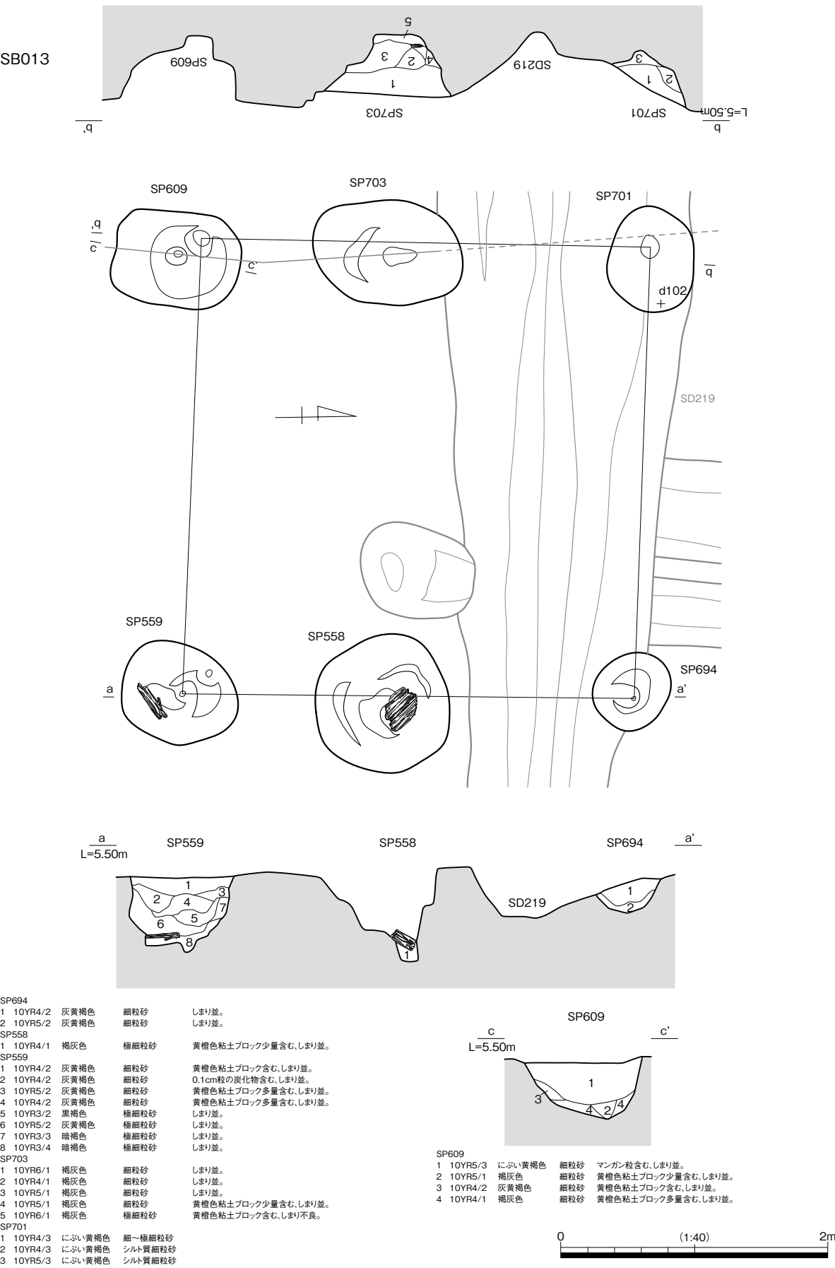
2b区 SB013 遺構図
