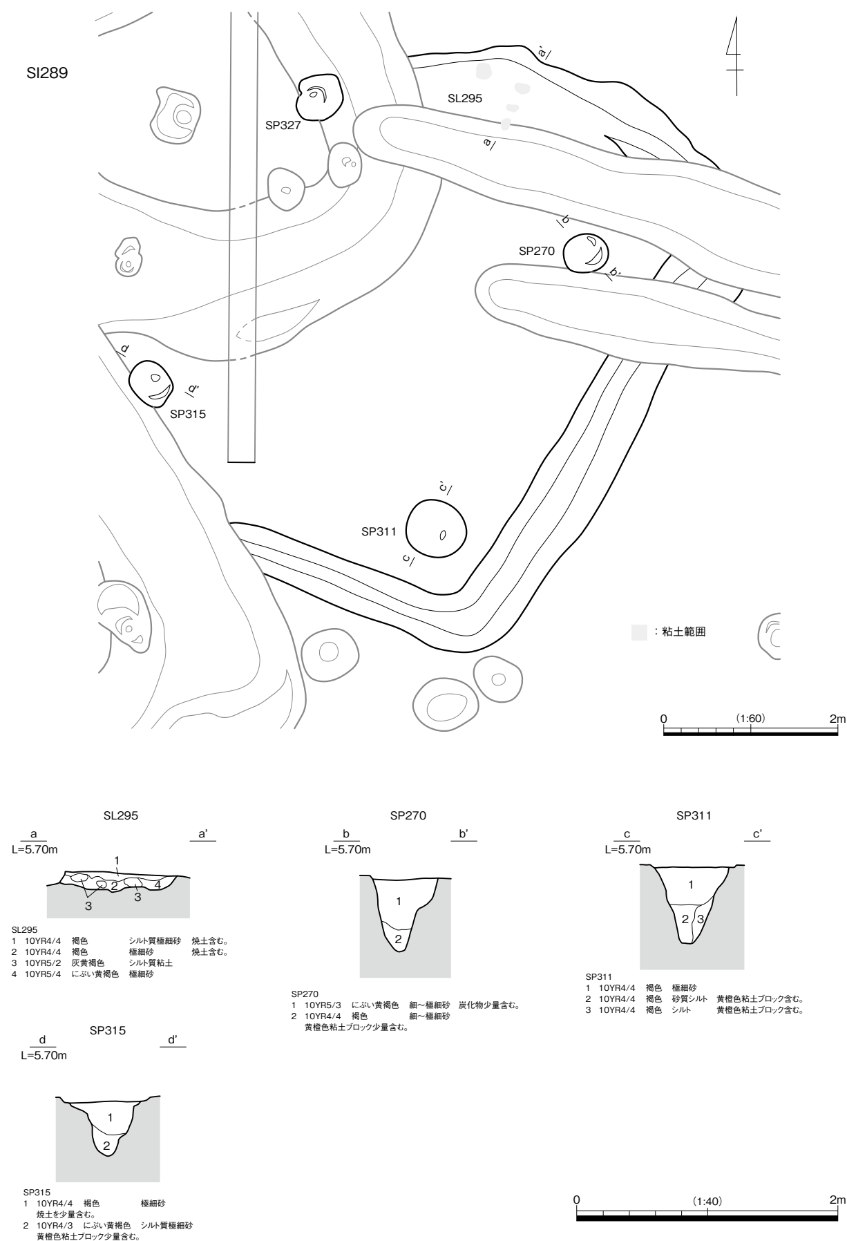
2b区 SI289 遺構図
