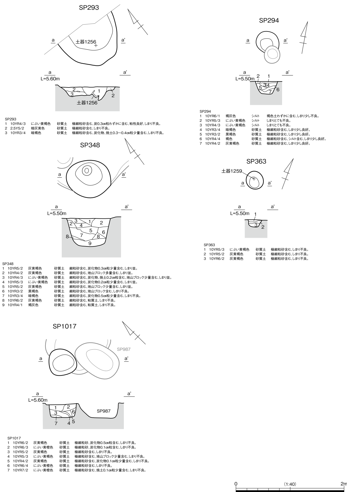
2c区 SP293・SP294・SP348・SP363・SP1017 遺構図
