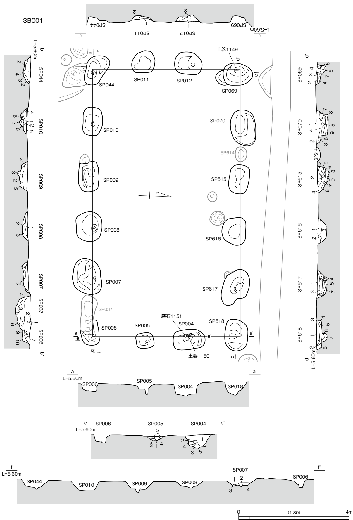
2c区 SB001① 遺構図
