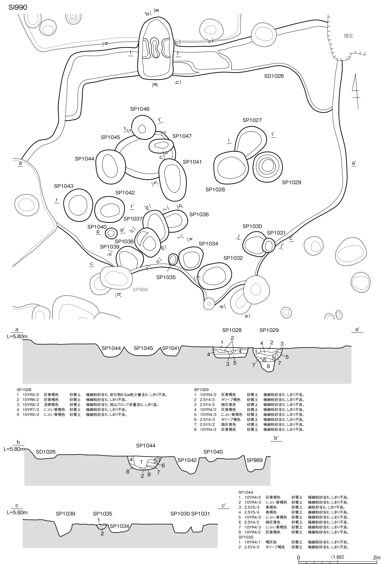
2c区 SI990① 遺構図
