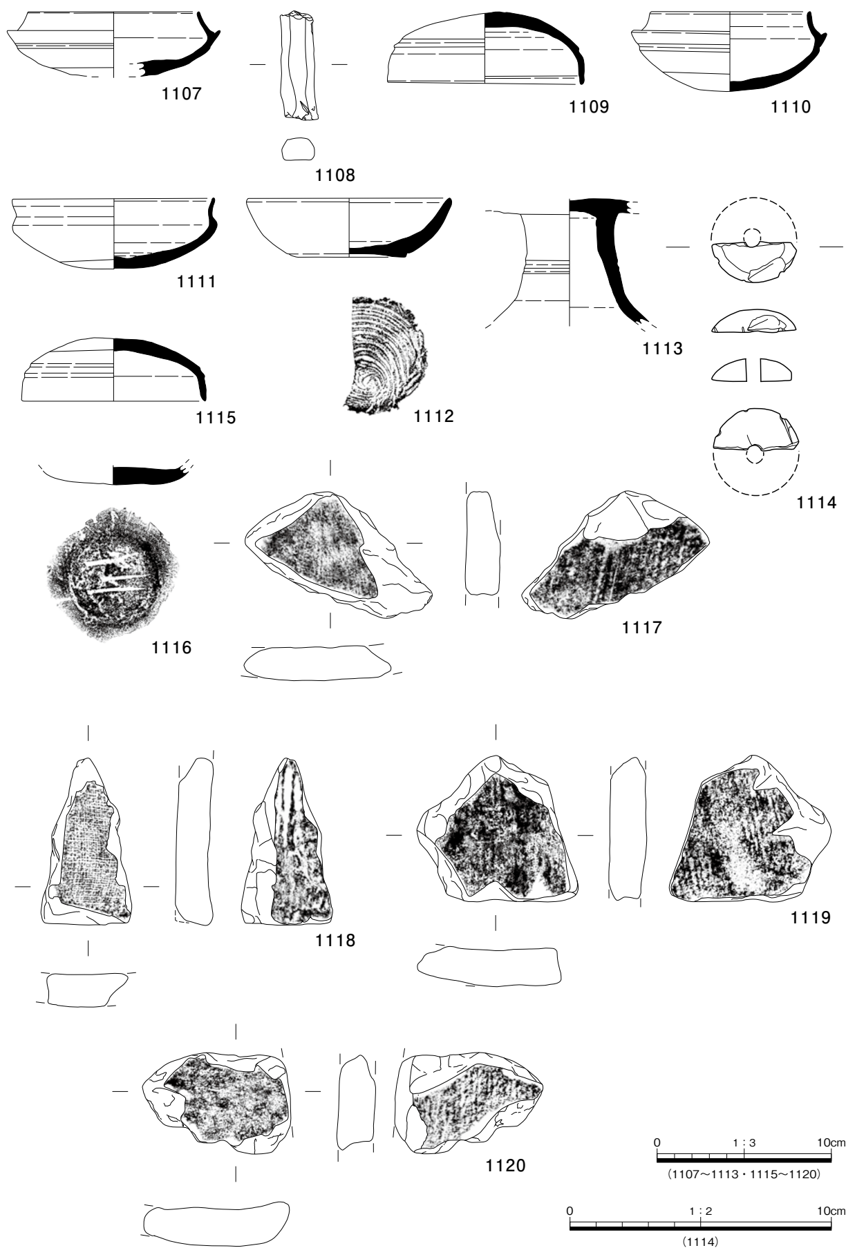
2b区 遺物実測図(12)
