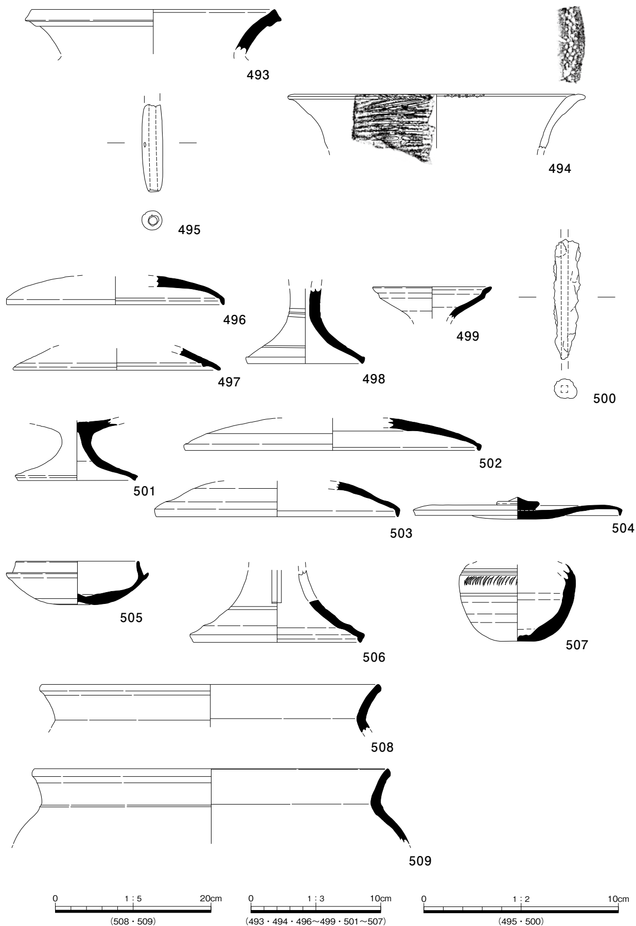
1d区 遺物実測図(1)
