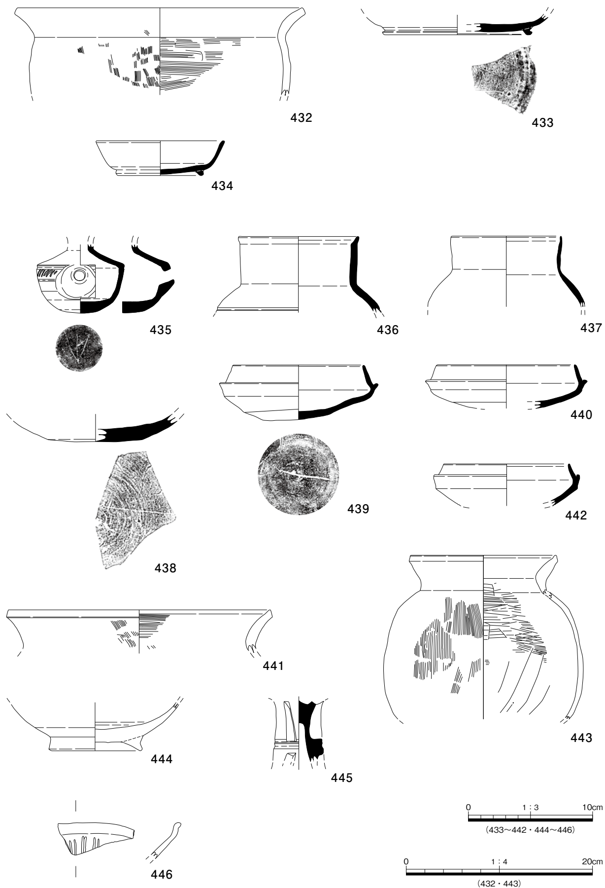
1c区 遺物実測図(17)
