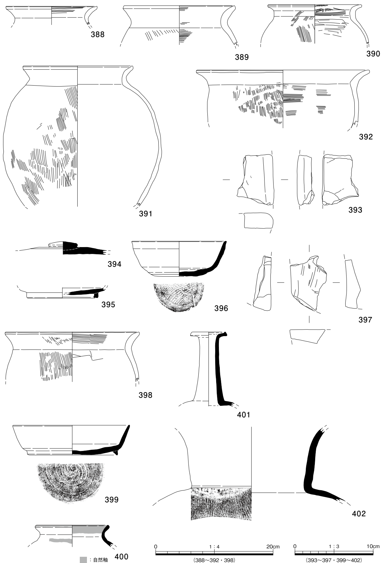
1c区 遺物実測図(14)
