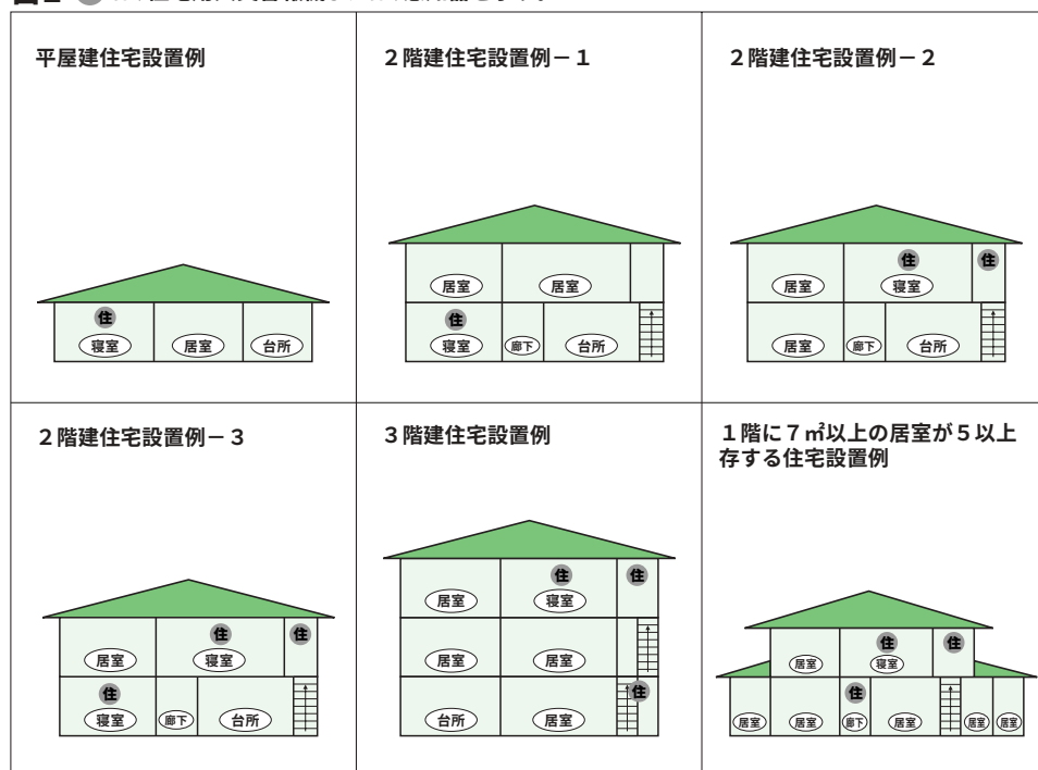
図1 住は、住宅用火災警報機または、感知器を示す。
